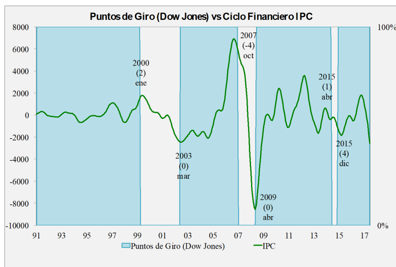
Figura 10. Fechado de los puntos de giro del DJ versus los ciclos del IPC, de noviembre de 1991 a abril de 2018, con las fechas de los puntos de giro del DJ determinadas con el algoritmo de B&B. Fuente: elaboración propia con información de Yahoo Finance.
