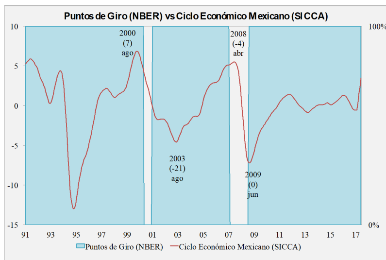
Figura 9. Fechado de los puntos de giro del NBER versus los ciclos del indicador coincidente del SICCA, las fechas señaladas son los puntos de giro del SICCA. Fuente: elaboración propia con información de INEGI y NBER.
